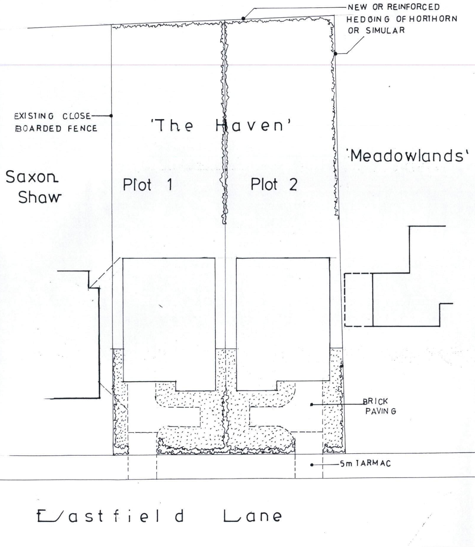
Site Plan 1:250
